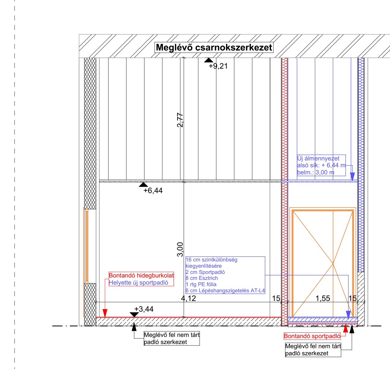
A-A METSZET M= 1:50
